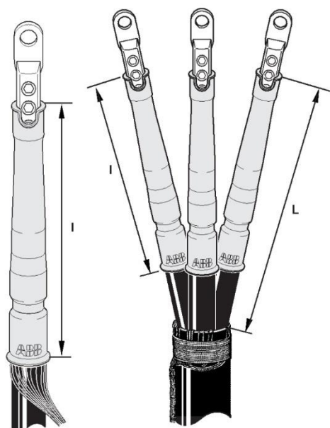
SOT внутренней установки
