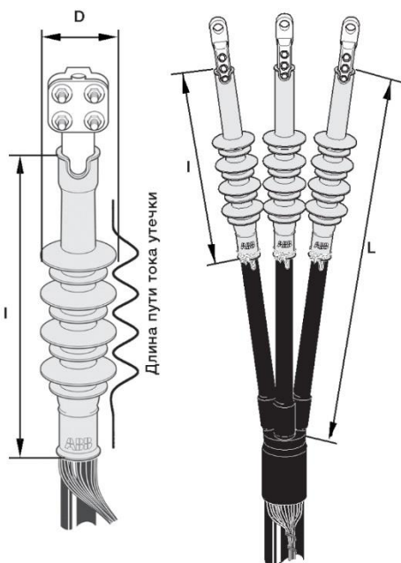
SOT наружной установки
