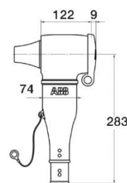
CSEP-A, 36-42 кВ, размеры 1-2
