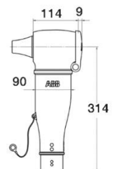
CSEP-A, 12-24 кВ, размер 3
