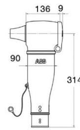
CSEP-A, 36-42 кВ, размер 3
